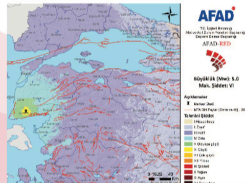
20 Şubat 2019 Ayvaık Çanakkale Depremi Tahmini Şiddet Haritası - AFAD-RED
